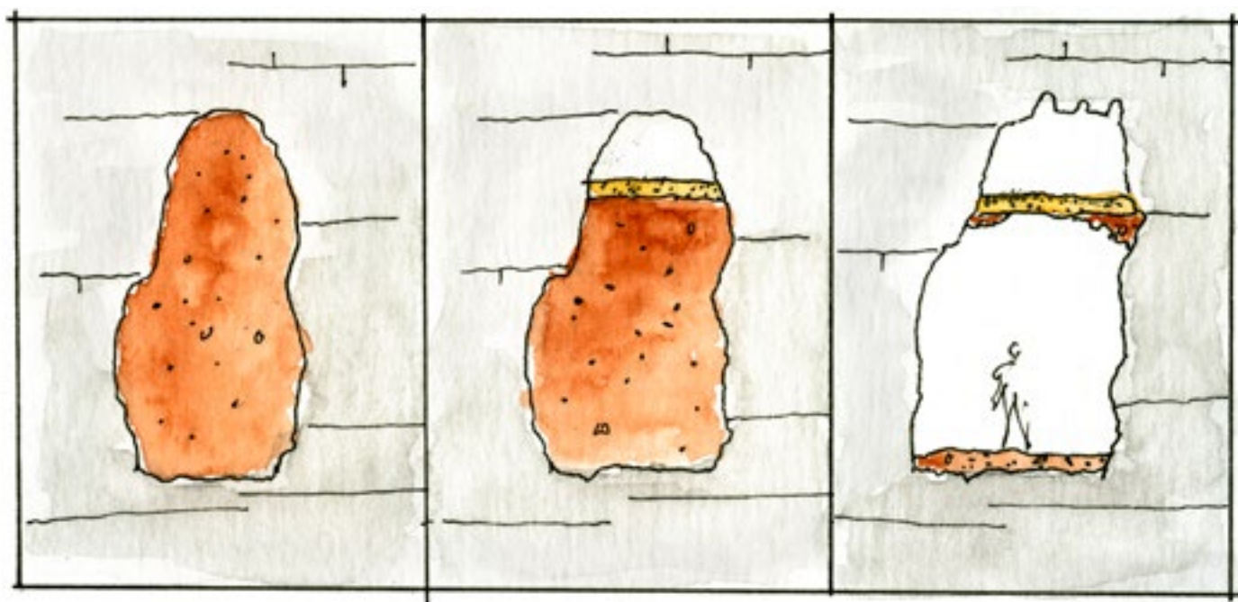
Sequência evolutiva de formação de paleopisos: (1) conduto preenchido por sedimentos, (2) remoção, da parte superior dos sedimentos, por água e deposição do paleopiso, (3) nova remoção, da parte inferior dos sedimentos, por água e permanência dos paleopisos, que formam capas mais resistentes. VM
